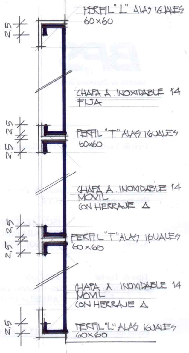
CORTE 1:5
