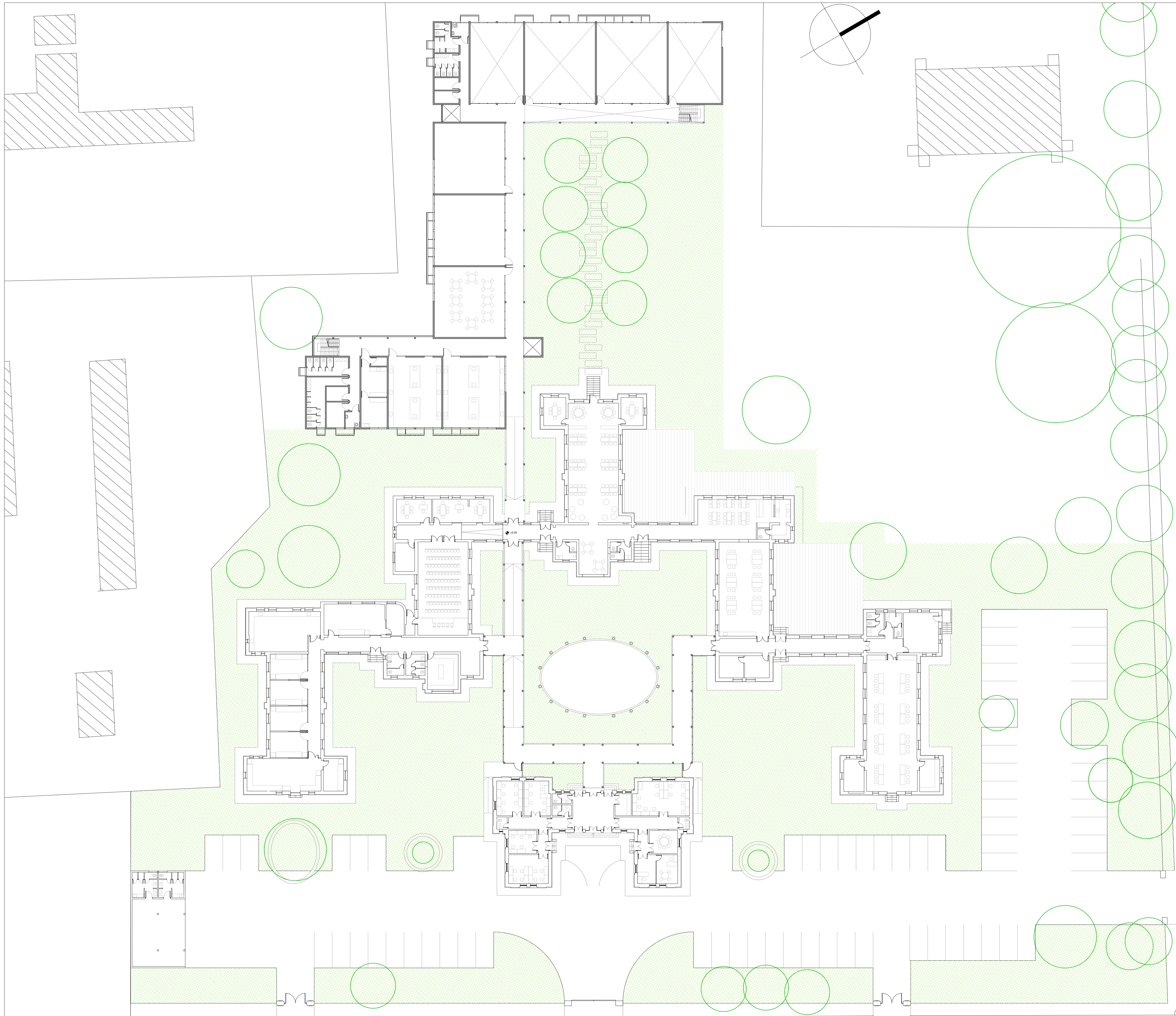
PLANTA BAJA esc. 1:250
